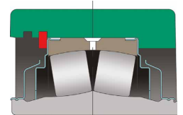
Labirent sızdırmazlık
